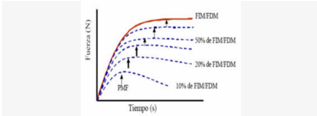
Figura 3. Valores de Fuerza Dinámica Máxima Relativa. (González y Gorostiaga, 2004). Cuando la carga es inferior a la FIM o la FDM, el PMF que se puede alcanzar será progresivamente menor
